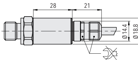
8252.XX.XXXX.22/24/88.XX.XX
