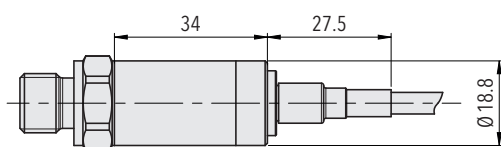
8252.XX.XXXX.08.XX.XX
