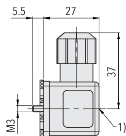
1) Torque de aperto 50 ... 60 Ncm
