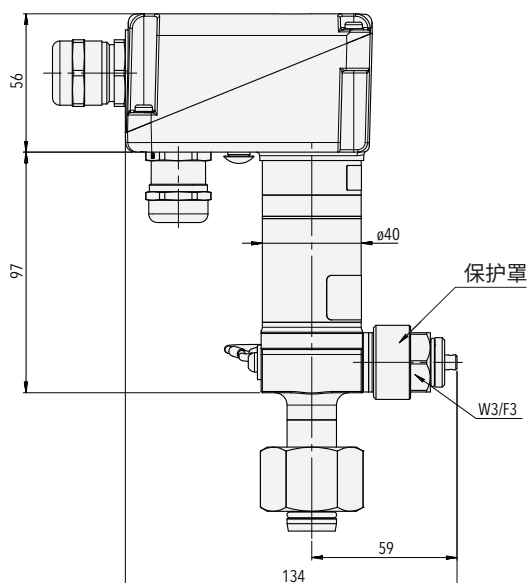
轴向连接的示例模型
