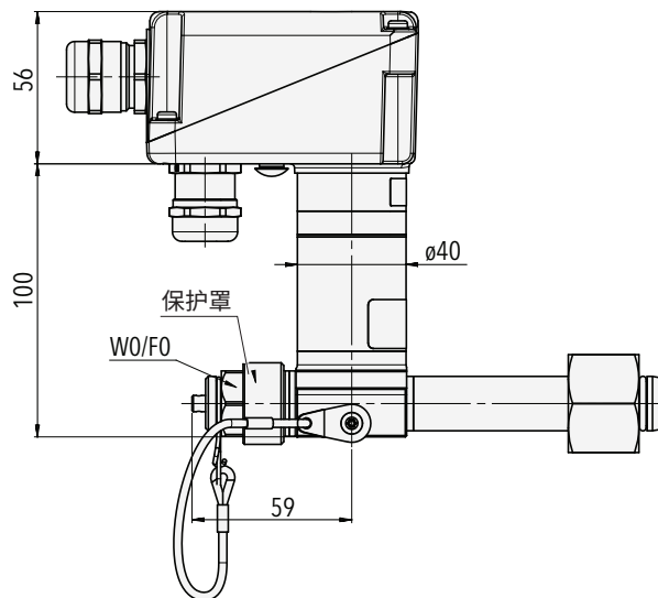
径向连接的示例模型
