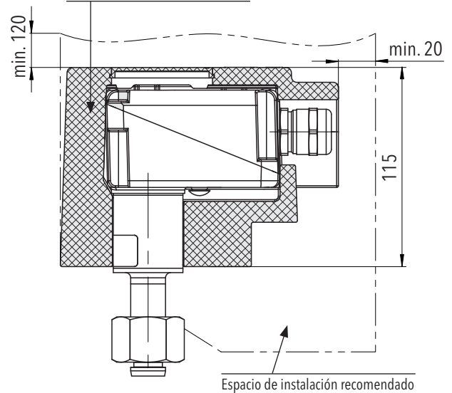
Cubierta de espuma térmica 87x6.XX.XXXX.XX.XX.XX.37
