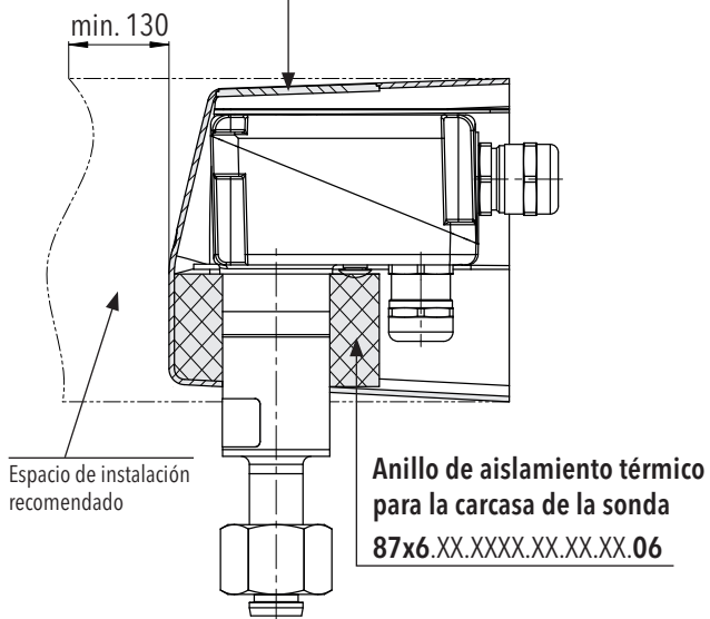
Cubierta de protección contra la intemperie 87x6.XX.XXXX.XX.XX.XX.46
