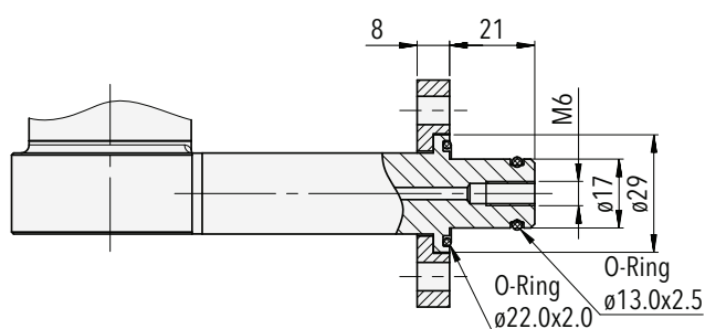
87x6.XX.2XP2.XX.XX.XX.XX Radial pour raccord bridé à deux trous
