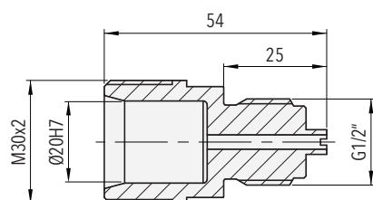
87x6.XX.2300.XX.XX.XX.N1 Adaptateur 2300 - G1/2" mâle pour raccord de pression G1/2" orientable
