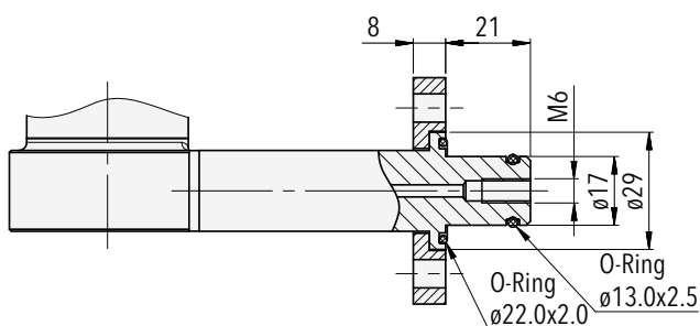
87x6.XX.2XP2.XX.XX.XX.XX Radiale per collegamento flangia a due fori
