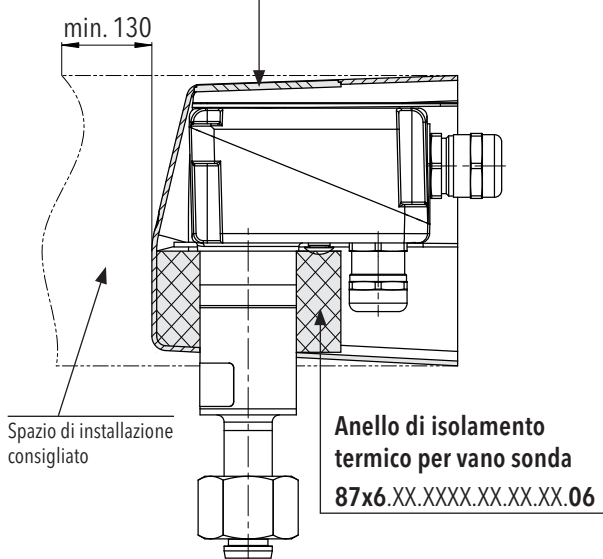
Copertura di protezione da agenti atmosferici 87x6.XX.XXXX.XX.XX.XX.46
