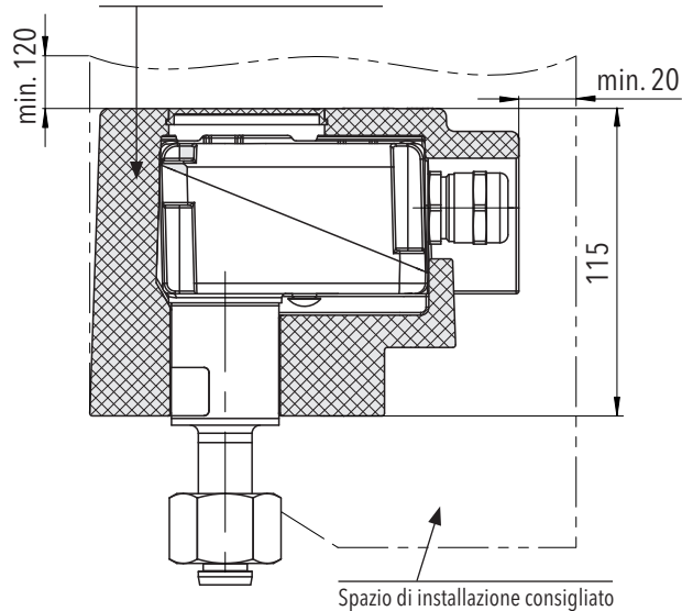
Copertura a schiuma termica 87x6.XX.XXXX.XX.XX.XX.37
