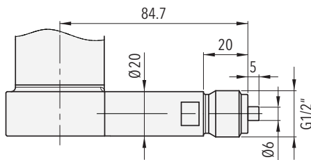
87x6.XX.1030.XX.XX.XX.XX Collegamento filettato radiale G1/2"
