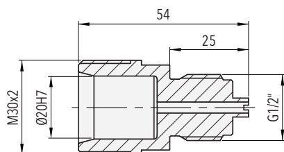
87x6.XX.2300.XX.XX.XX.N1 Adattatore 2300 - maschio G1/2" per collegamento a pressione G1/2" girevole
