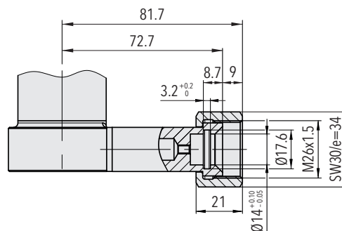
87x8.XX.2XE2.XX.XX.XX.XX ラジアル接続 DN8
