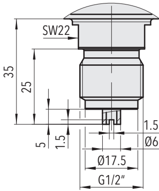
87x8.XX.1000.XX.XX.XX.XX 軸方向ねじ接続 G1/2"
