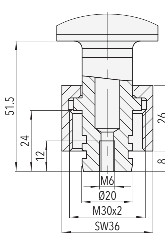
87x8.XX.2300.XX.XX.XX.XX 軸方向袋ナット接続
