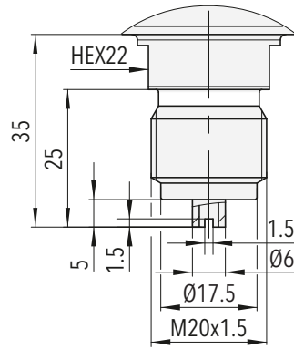
87x8.XX.1120.XX.XX.XX.XX 軸方向ねじ接続 M20x1.5
