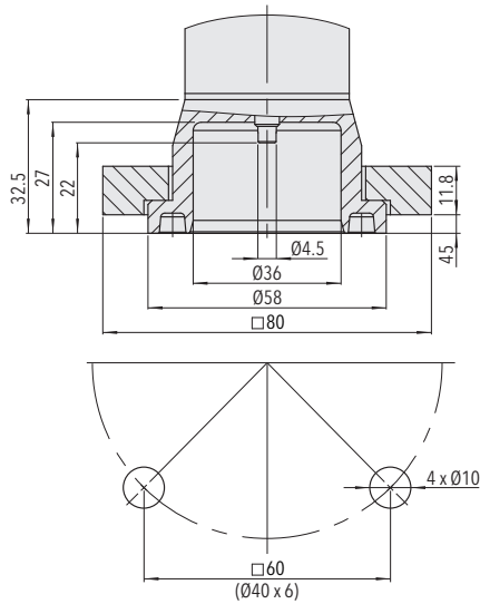
87x8.XX.2000.XX.XX.XX.XX 軸フランジ接続
