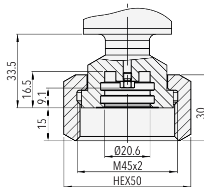
87x8.XX.2570.XX.XX.XX.XX 接続の軸 DN20
