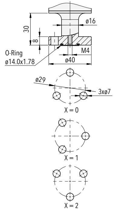
87x8.XX.220x.XX.XX.XX.XX 軸フランジ接続
