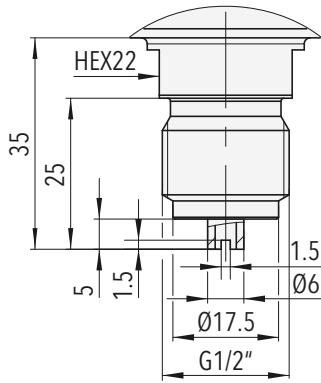
87x8.XX.1000.XX.XX.XX.XX 軸方向ねじ接続 G1/2"
