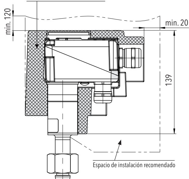
Cubierta de espuma térmica 878x.XX.XXXX.XX.XX.XX.37
